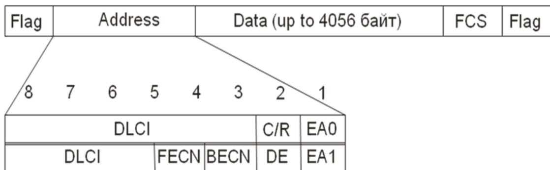
Рисунок 2.1.2 – Формат кадра Frame Relay
