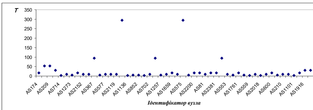
Рисунок 6.1.2 – Розподіл вузлів за метрикою довіри. Вісь ординат – метрика довіри в формі 10^{T_u}
