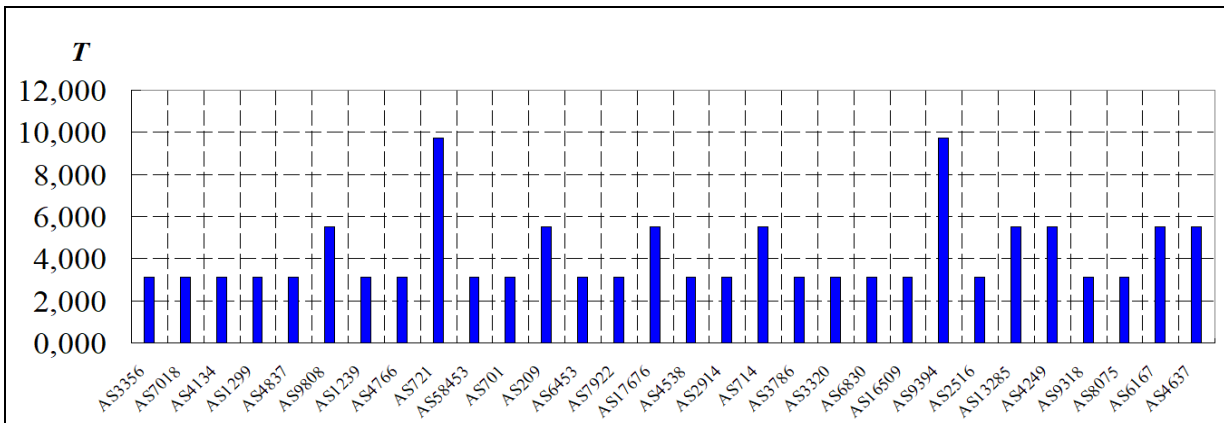
Рисунок 6.2.3 – Розподіл вузлів за метрикою довіри. Вісь ординат – метрика довіри в формі 10^{T_u^v}
