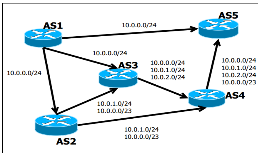
Рисунок 4.1.1 – Графічна модель експорту анонів IP-префіксів в процесі взаємодії 5 автономних систем
