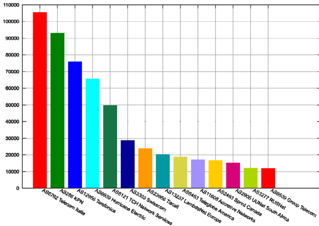
Рисунок 3.2.3 – Кількість ретрансльованих хибних префіксів (вісь ординат) через інші AS (вісь абсис). Джерело даних – MERIT
