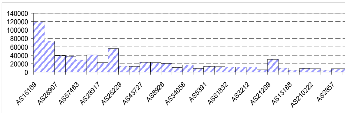
Рисунок 6.3.3 – Графік розподілу ризику серед 100 AS з максимальною метрикою значущості. Збережено впорядкування за значенням метрики значущості. Вісь ординат – ризик R
