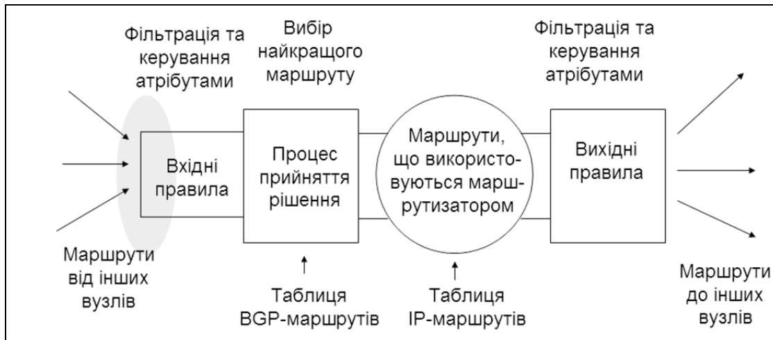
Рисунок 1.2.1 – Функціональна схема протоколу маршрутизації BGP-4
