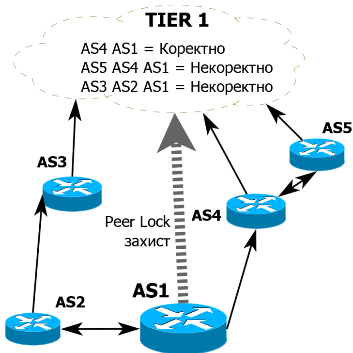
Рисунок 1.4.3 – Схема взаємодії операторів із застосуванням механізму Peer Lock
