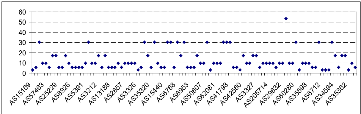
Рисунок 6.3.2 – Графік розподілу за метрикою довіри серед 100 AS з максимальною метрикою значущості. Вісь ординат – метрика довіри в формі 10^{T_u^v}
