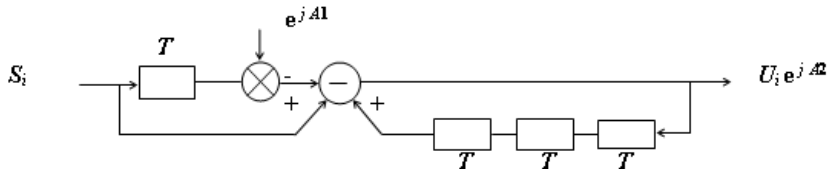
Рис. 4. Обчислення згідно (7)
