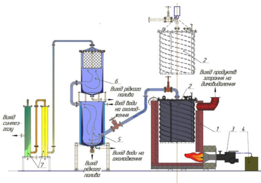
Рисунок 1 – Схема установки утилізації відходів
