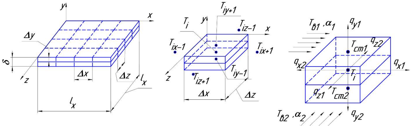
Рис. 4. Поділ теплообмінника на розрахункові елементи
