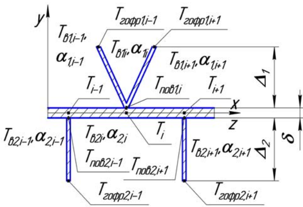
Рис. 2. Схема теплопередаючих пластин
